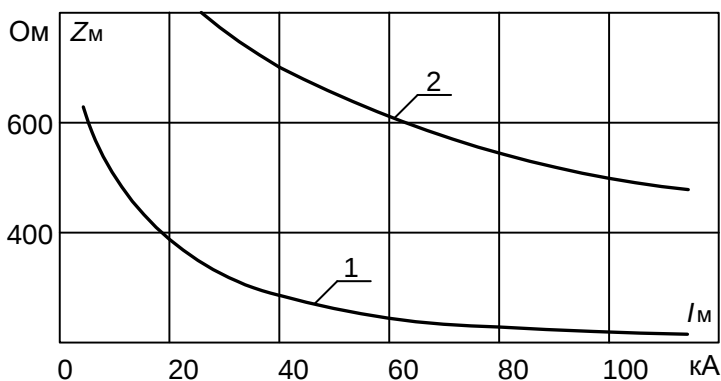
Рис. 1. Зависимость волнового сопротивления канала от тока: 1 – по данным [3]; 2 – по данным [1].
