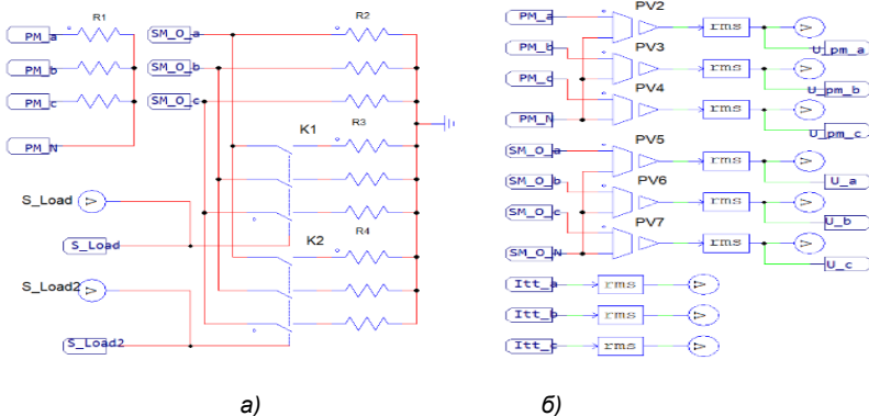
Рис. 3. а) модели нагрузки, б) модель блока измерений
