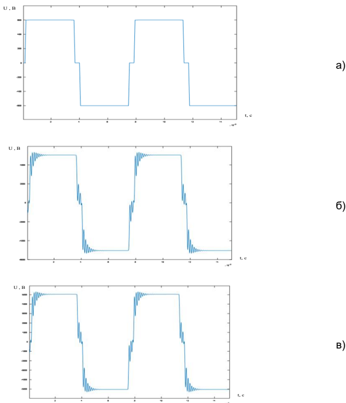
Рис. 4. Расчетные осциллограммы напряжения: ЭДС транзисторного преобразователя (а), напряжения в начале высоковольтной кабельной линии (б), напряжения в конце высоковольтной кабельной линии (в)
