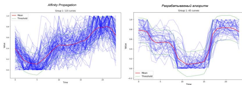
Рис. 3. Первый набор профилей нагрузки, полученных алгоритмом Affinity Propagation и разрабатываемым алгоритмом
