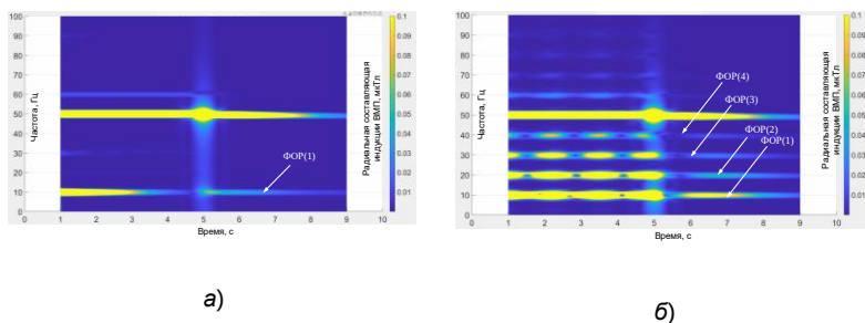
Рис. 1. ЧВС ВМП АД типа ДАЗО2-17-44-8/10У1 в режиме выбега: а – исправная обмотка ротора; б – обмотка ротора с одним оборванным стержнем
