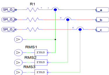
Рис. 4. Модель фидера ТСГ и БДТ
