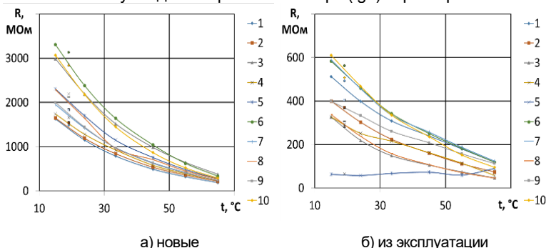
Рис. 2. Температурная зависимость сопротивления варисторов УЗИП
