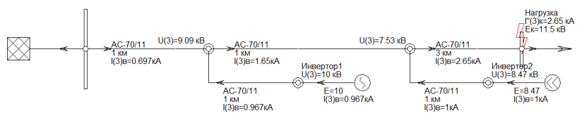
Рис. 3. Результаты расчета на второй итерации выбора режима
