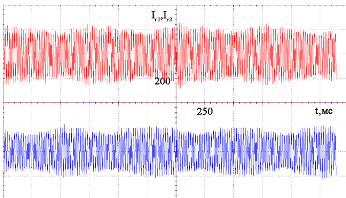
Рис. 1. Обменные колебания мощности
