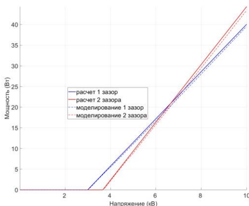
Рис. 3. Зависимость мощности разряда от напряжения на генераторе озона
