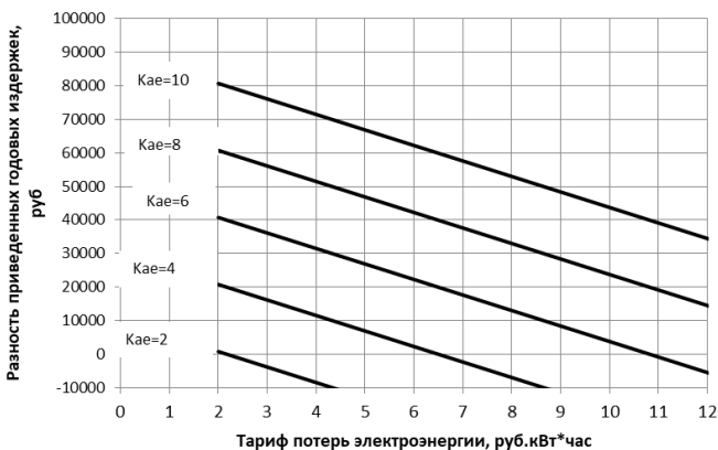
Рис. 1 Разность приведенных эксплуатационных издержек сравниваемых трансформаторов
