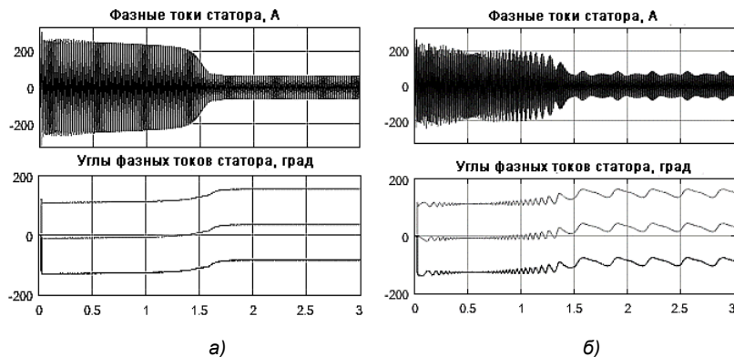
Рис. 1. Результаты компьютерного моделирования работы асинхронного электрического двигателя: а) при исправной обмотке ротора; б) при обрыве четырех стержней обмотки ротора
