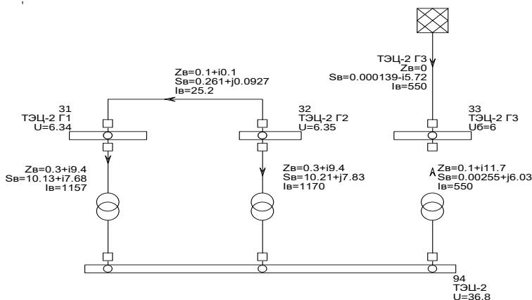
Рис.3 Расчет с учетом АЧР I и АЧР- II f = 49,8 Гц
