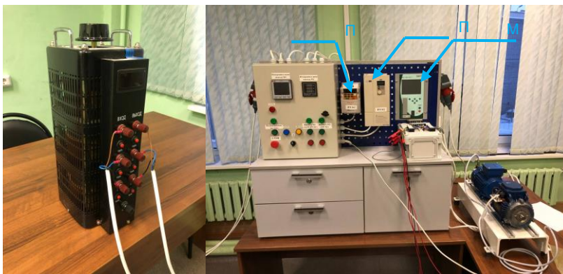
Рис.2. Общий вид стенда, ЛАТР (слева)
