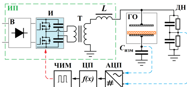
Рис.1 Блок-схема ГО с системой управления источника питания
