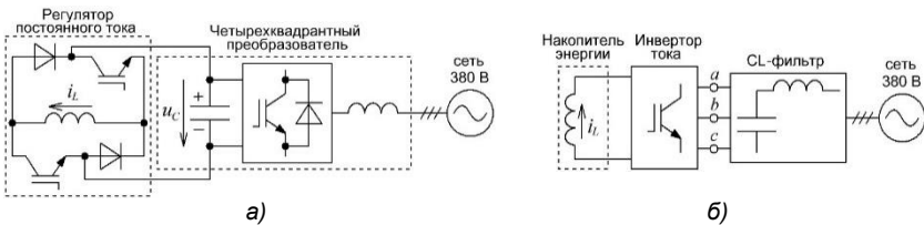
Рис. 1. Структурные схемы регулятора мощности на базе индуктивного накопителя: а – на основе преобразователя напряжения и регулятора постоянного тока; б – на основе преобразователя тока с выходным CL-фильтром
