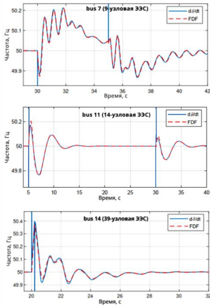
Рис. 1. а – расширение состава переменных физического соединения и описания модели линии электропередачи на языке Simscape; б – примеры динамики изменения узловой частоты
