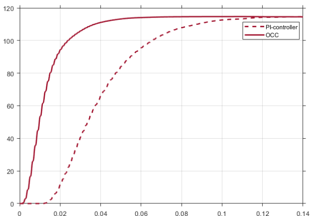
Рис. 2. Стабилизация действующего значения напряжения от времени
