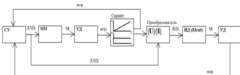
Рис. 2. Схема модели САУ в Simulink
