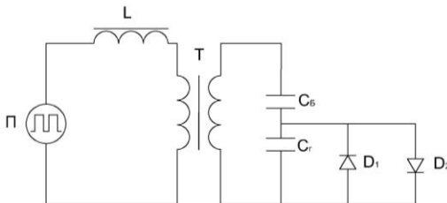
Рис. 2. Общая схема замещения барьерного озонатора
