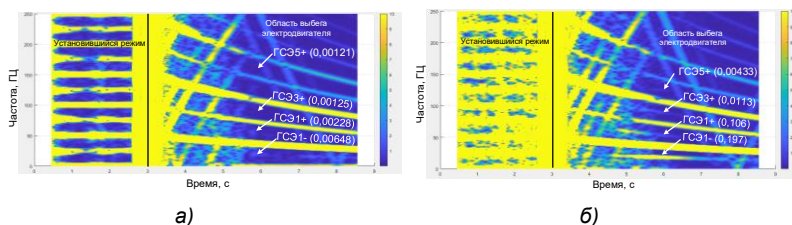
Рис. 3 – Спектры ВМП АД при отсутствии СЭ (а) и с наличием 30% СЭ (б) в режиме выбега (в скобках указаны амплитуды гармоник в мкТл)
