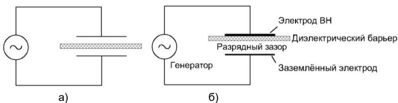
Рис. 1. Модель озонатора: двойной (а) и одинарный зазор (б)
