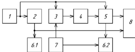
Рис. 2. Структурная схема модели проверки характеристик ТСГ
