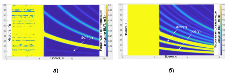
Рис. 2. ЧВС ВМП АД типа АИР 71А6 в режиме выбега: а – исправная обмотка ротора; б – обмотка ротора с одним оборванным стержнем
