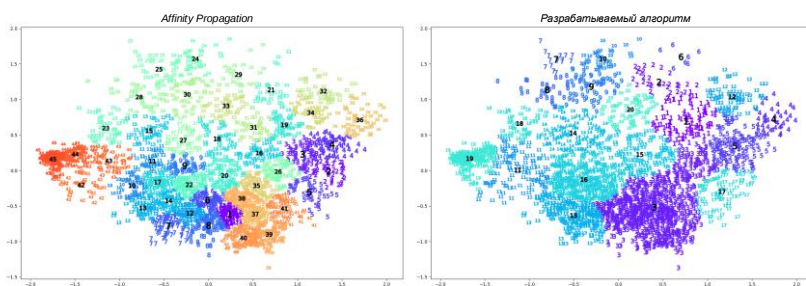
Рис. 2. Карты кластеров на двухмерной плоскости
