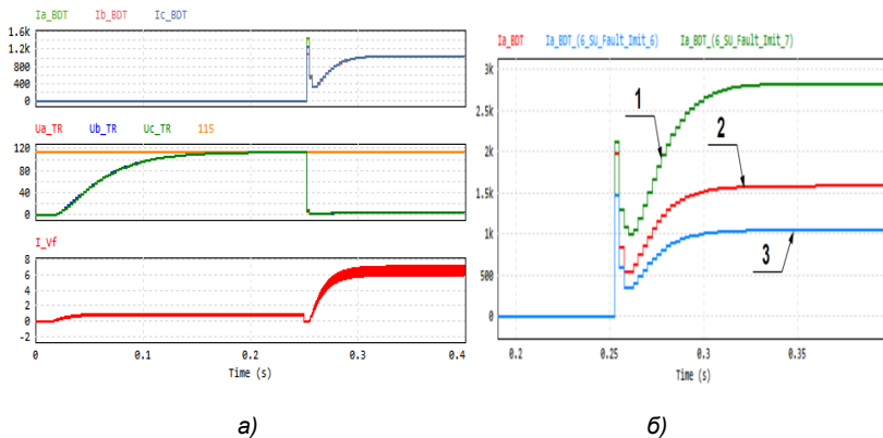
Рис. 8. Временные диаграммы процессов в КГ при аварийных режимах
