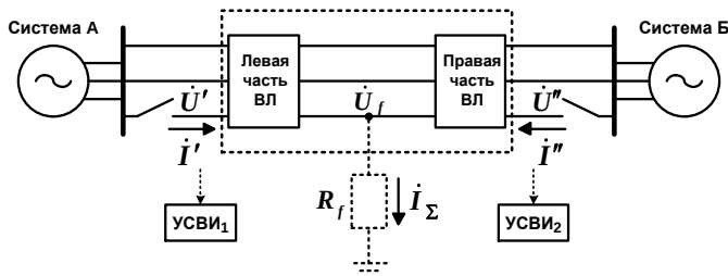
Рис. 1. Иллюстрация к организации СВИ по концам ВЛ СВН при самоустранении однофазного КЗ в течение БП ОАПВ
