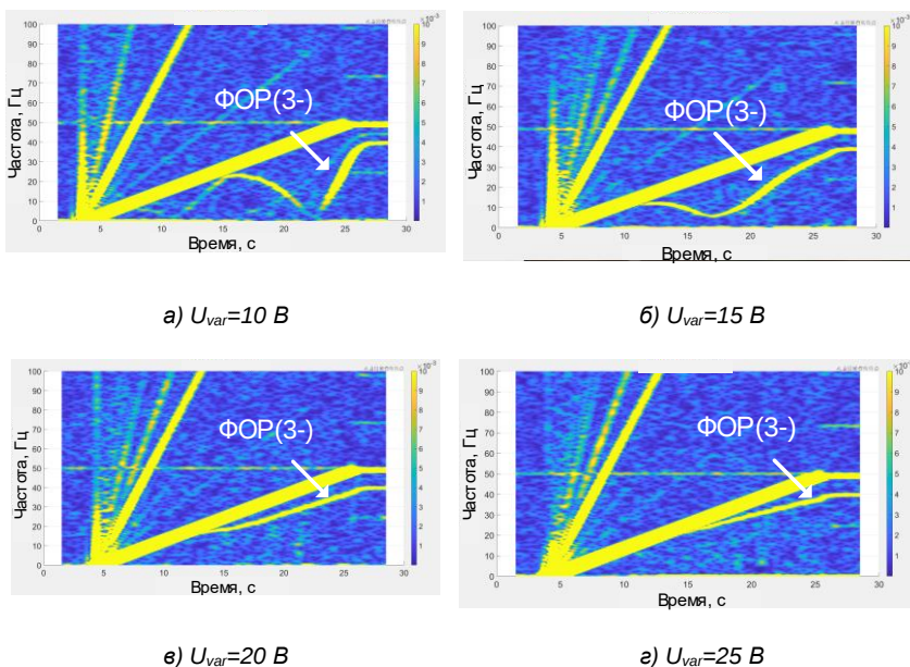
Рис. 2. ЧВС сигналов тока статора при наличии оборванного стержня обмотки ротора при различных значения параметра U_{var}
