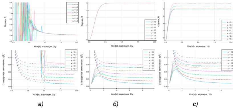
Рис. 1. Статистические испытания оценок ( R = 5 \text{ Ом} ): а – (6), б – (10), с – (9)
