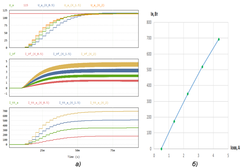
U_a – выходное напряжение ТСГ, I_{Vf} – ток возбуждения, I_{tt} – выходной ток ТСГ Рис. 5 а) токи и напряжения исследуемой модели, б) регулировочная характеристика ТСГ
