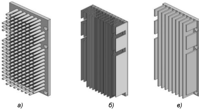
Рис. 4. Рассматриваемые варианты радиаторов
