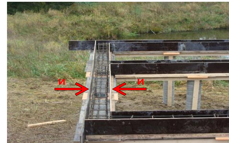
И – поверхности опалубки для установки индукторов
