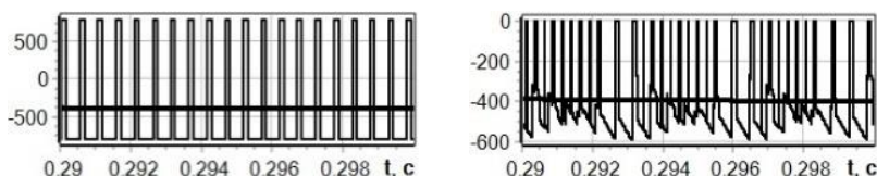
Рис. 4. Диаграммы напряжения на накопителе (половина периода): слева – в схеме с инвертором напряжения; справа – в схеме с инвертором тока
