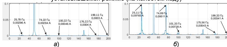
Рис. 2. Спектры тока статора АД при отсутствии СЭ (а) и при наличии 30% СЭ (б) в установившемся режиме (на холостом ходу)
