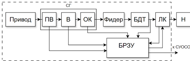
Рис. 1. Структурная схема канала генерирования
