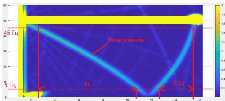
Рис. 2. Спектрограмма сигнала двигателя с одним оборванным стержнем ротора с указанием зон используемых для срабатывания
