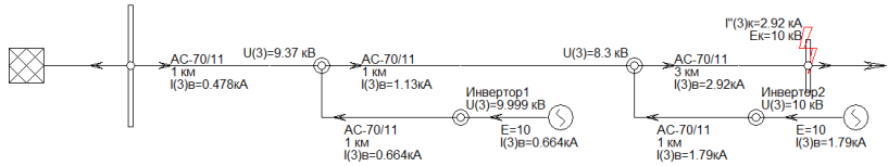
Рис. 2. Результат расчета, в предположении, что инверторы в режиме стабилизации напряжения
