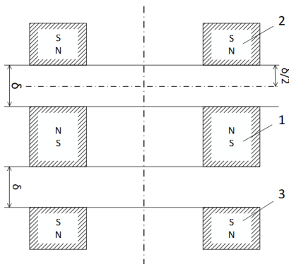
Рис. 1. Магнитный подвес магнитоожидкостного датчика вибродиагностики: 1 – чувствительный элемент; 2,3 – постоянные магниты магнитного подвеса
