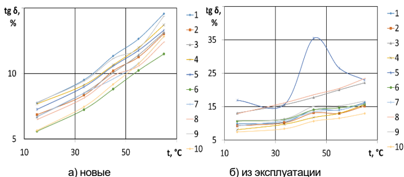
Рис. 3. Температурная зависимость тангенса угла диэлектрических потерь УЗИП
