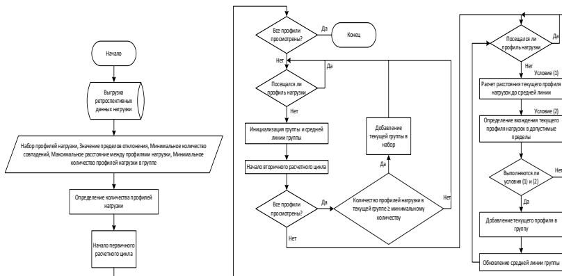
Рис. 1. Блок-схема разрабатываемого алгоритма группирования профилей нагрузки
