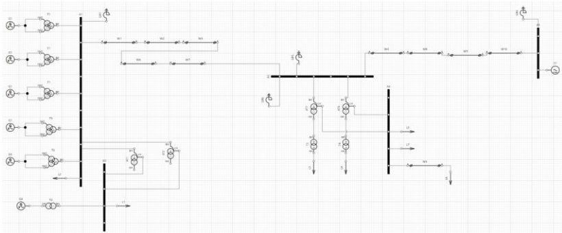
Рис. 1. Общий вид одной из моделей ЭЭС в сервисе «Лаборатория РЗА»
