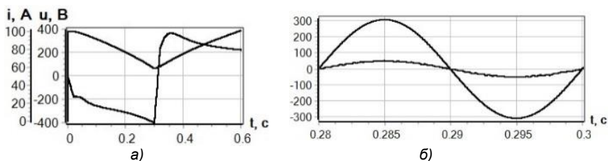
Рис. 3. Результаты моделирования регулятора на основе преобразователя тока: а – диаграммы постоянной составляющей напряжения и тока накопителя; б – диаграммы тока и напряжения сети для фазы А (один период)
