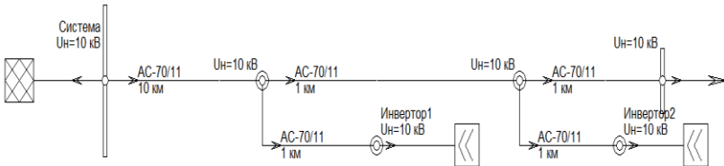
Рис. 1. Исходная схема в ПО СИМЭС для тестирования подхода
