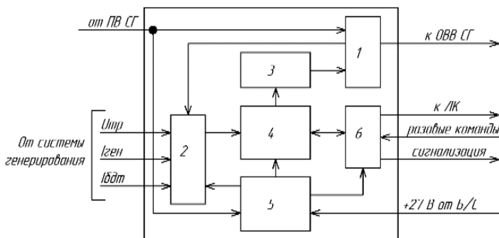
Рис. 1. Структурная схема блока
