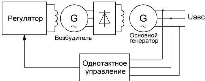
Рис. 1. Структурная схема управления синхронного генератора
