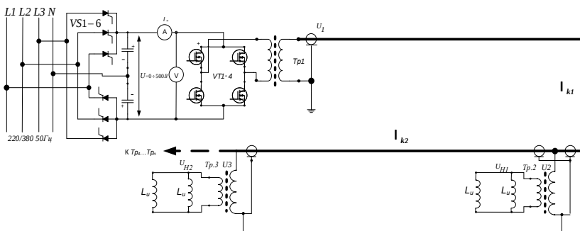
Рис. 3. Магистральная схема высоковольтного промышленного электроснабжения индукторов при ЭТО свайно-ростверковых фундаментов:
