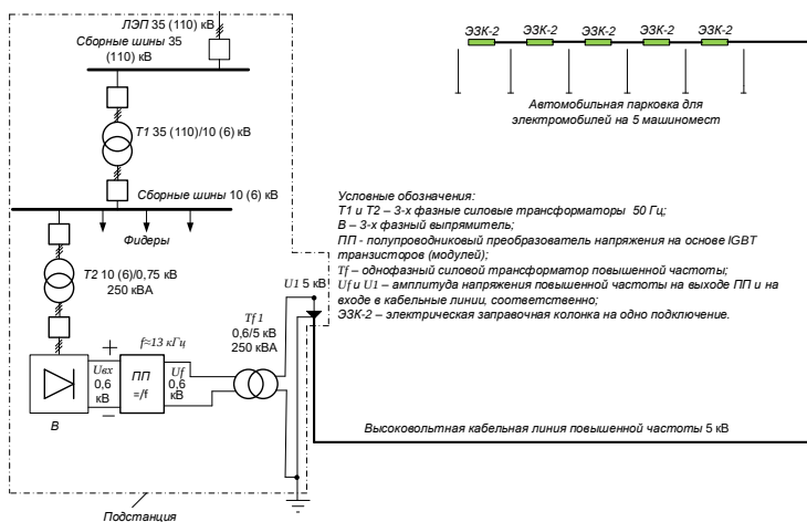
Рис. 4. Общая схема варианта системы электроснабжения повышенной частоты зарядных станций 6 автомобилей одновременно мощностью 200÷250 кВА
