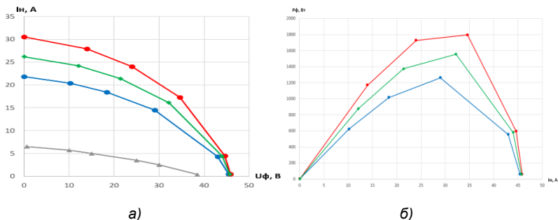
Рис. 4. а) внешняя характеристика ПВ, б) кривая электромагнитной мощности ПВ
