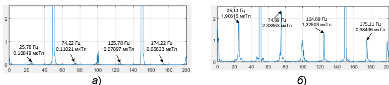
Рис. 1. Спектры ВМП АД при отсутствии СЭ (а) и при наличии 30% СЭ (б) в установившемся режиме (на холостом ходу)
