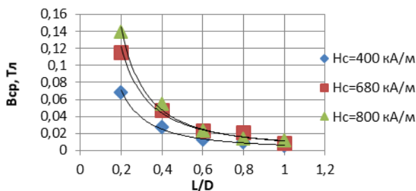
Рис. 2. Зависимость средней индукции от расстояния между чувствительным элементом и одним из магнитов магнитного подвеса
