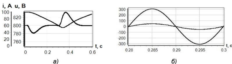
Рис. 2. Результаты моделирования регулятора на базе инвертора напряжения: а – диаграммы напряжения на конденсаторе и тока накопителя; б – диаграммы тока и напряжения сети для фазы А (один период)
