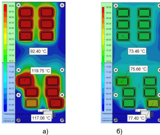
Рис. 5. Картины распределения температур по элементам СЧ
