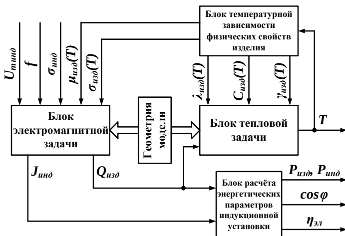
Рис. Структурная схема электротепловой модели индукционной установки
