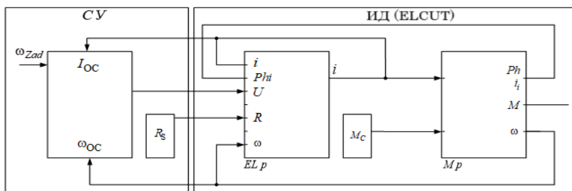
Рис. 1. Модель САУ синхронного привода с исполнительным двигателем на базе программного комплекса ELCUT, с реализацией в среде Simulink
