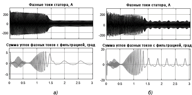
Рис. 2. Результаты компьютерного моделирования работы асинхронного электрического двигателя: а) при обрыве одного стержня обмотки ротора; б) при обрыве четырех стержней обмотки ротора
